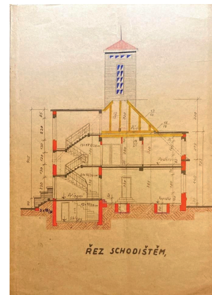
Obrázek 17 Vybraný plán z původních plánů zbrojnice.
