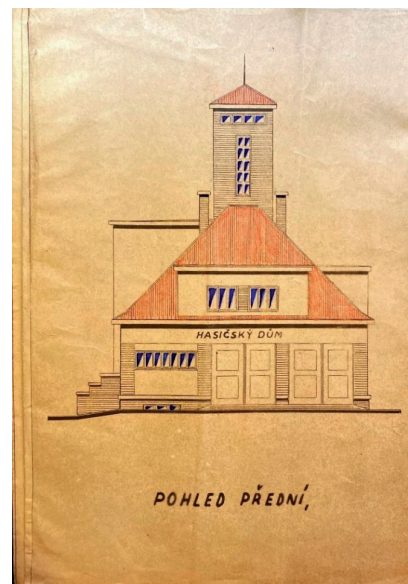
Obrázek 16 Vybraný plán z původních plánů zbrojnice.
