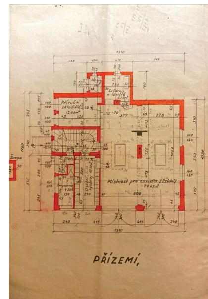
Obrázek 19 Vybraný plán z původních plánů zbrojnice.
