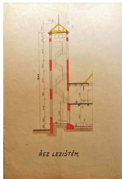
Obrázek 18 Vybraný plán z původních plánů zbrojnice.
